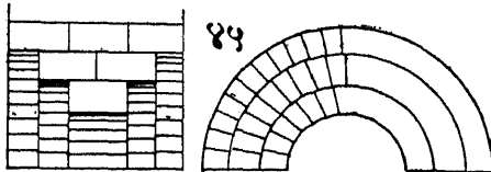
४५. Ordered arch : (विटांची) संयुक्त
